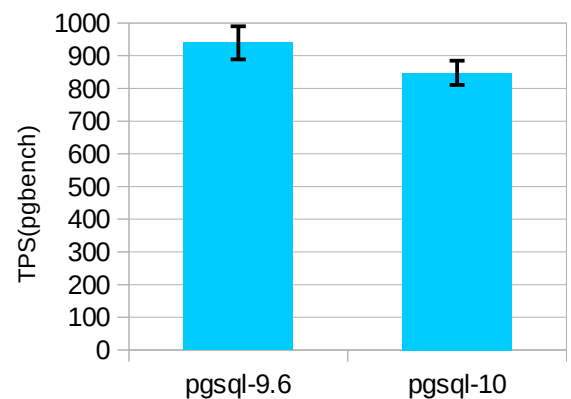
hash インデックス単一挿入
