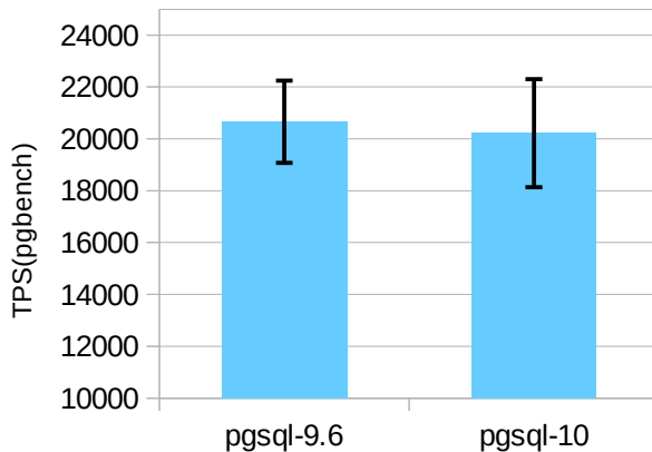
hash インデックス並列挿入
